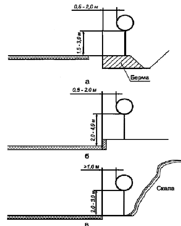
Рисунок В.1 - Типовое размещение знаков в поперечном профиле дороги: а - вне населенных пунктов; б - в населенных пунктах; в - на обочине в стесненных условиях
